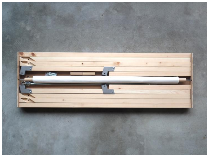
組立式マルシェ屋台「misekko」(収納時)
